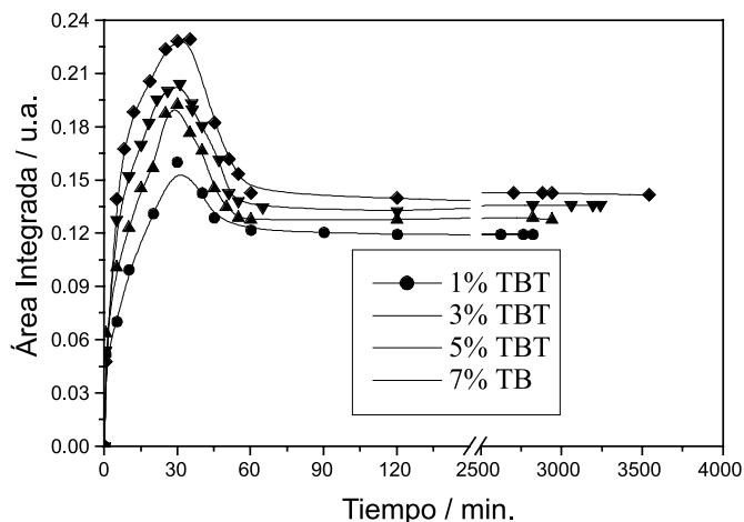
Figura 8. Evolución del área integrada de la banda situada a 936\text{ cm}^{-1} para todas las muestras estudiadas y para diferentes concentraciones de TBT.
